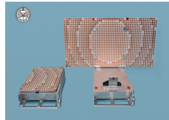
X-band HGA Reflectarray
